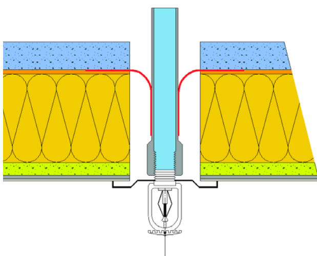
lufttæt (dampspærretape - rød)
